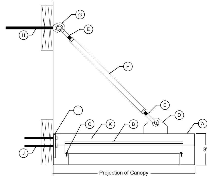
3 PROFILE SCALE: 1" = 1'-0"
