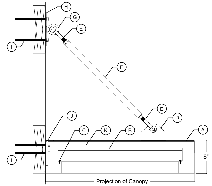
3 PROFILE SCALE: 1" = 1'-0"
