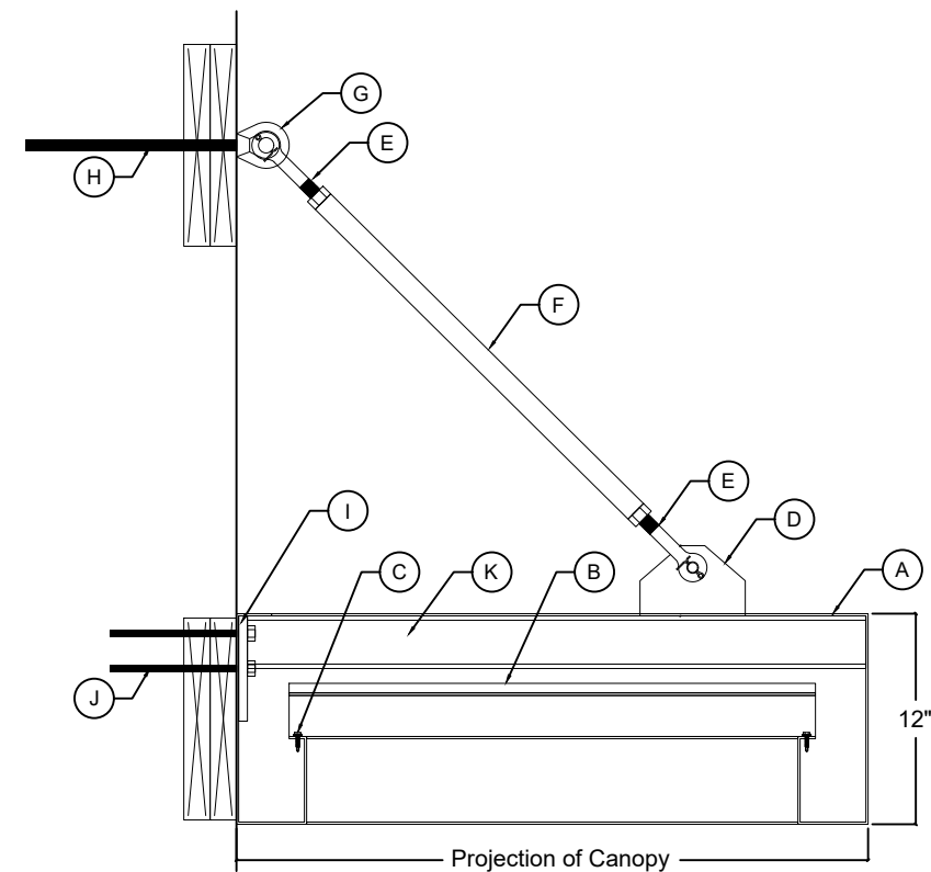
3 PROFILE SCALE: 1" = 1'-0"
