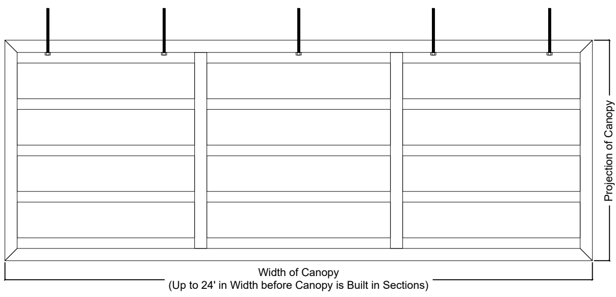
2 TOP VIEW SCALE: 3/4" = 1'-0"
